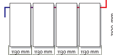
Einbaumaße tecSol
